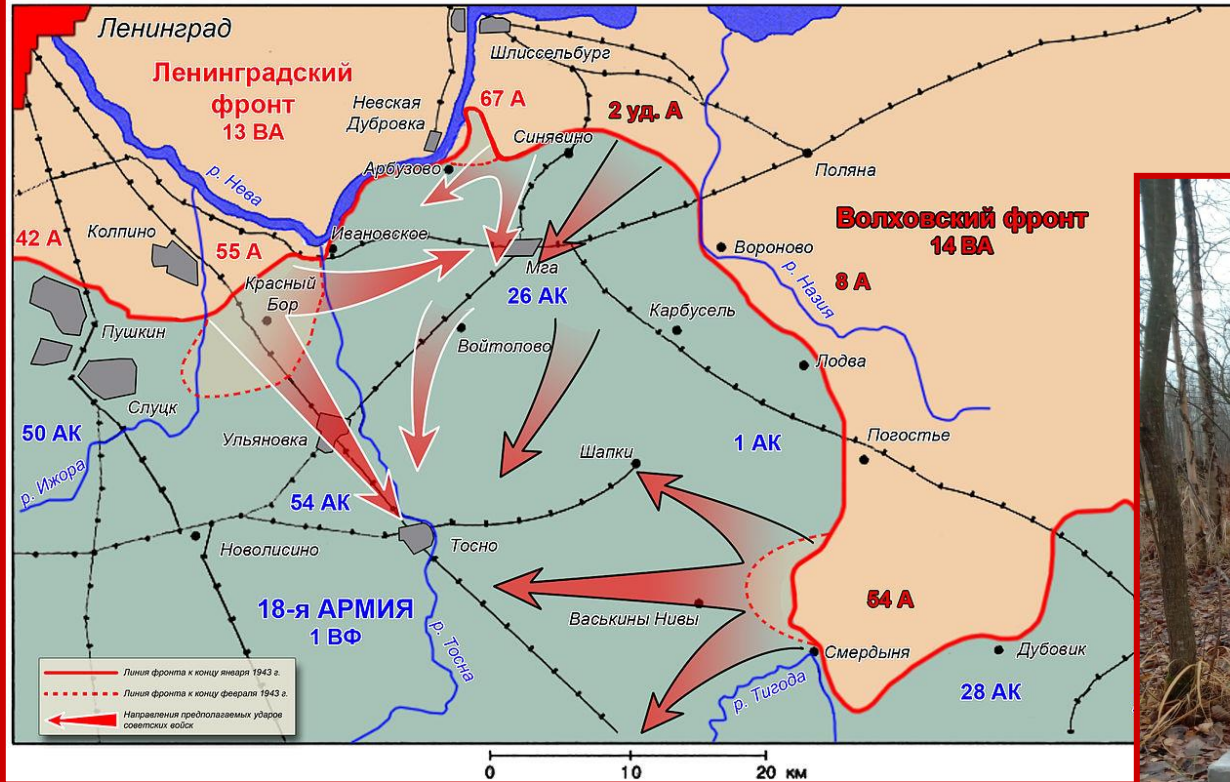
План наступления советских войск под Ленинградом в феврале 1943 г. (согласно директиве Ставки ВГК №30034 от 1 февраля 1943 г.)
